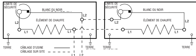
Figure 5 : Schémas de câblage
