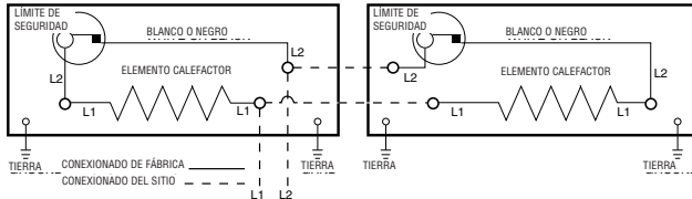
Figura 5: Diagramas de conexión
